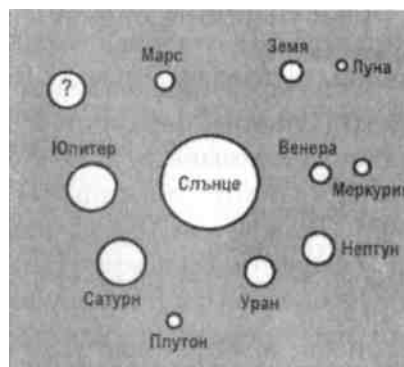
Изображение 29: За сравнение: нашата Слънчева система плюс една допълнителна, непозната планета.
