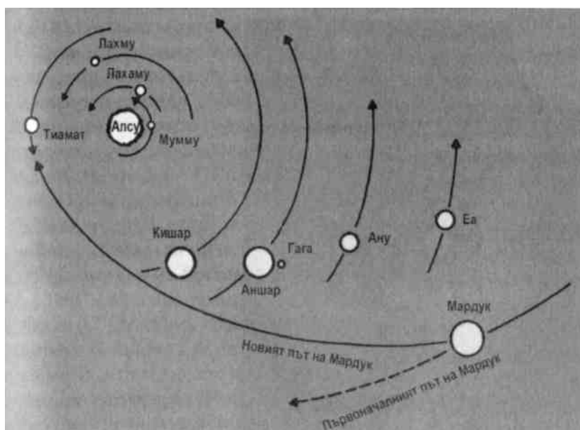
Изображение 31: Планетата Нибиру/Мардук прониква в Слънчевата система, бива привлечена от Слънцето и така се отклонява от първоначалната си орбита.
