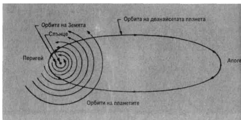
Изображение 30: Планетата Нибиру /Мардук обикаля Слънцето веднъж на всеки 3600 години.
