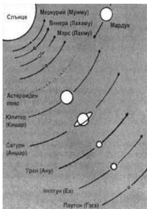
Изображение 33: Другата разрушена част на Тиамат е астероидният пояс, който днес се намира между Марс и Юпитер.
