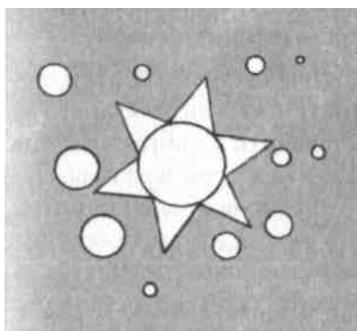
Изображение 28: Рисунокът върху ролковия печат показва още една допълнителна планета в нашата Слънчева система.
