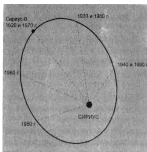
Изображение 49: Съвременна диаграма на орбитата на Сириус-В. Данните за годините се отнасят до позициите, които Сириус-В е заемала през тези периоди. Догоните не поставят Сириус-В в центъра на своята рисунка, а го разполагат близо до един от фокусите на елипсовидното образувание - изумителен детайл, който са знаели още преди 700 години!
