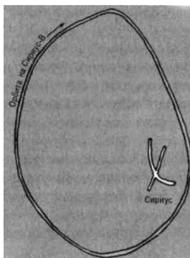
Изображение 48: Орбитата на Сириус-В според рисунка на догоните.
