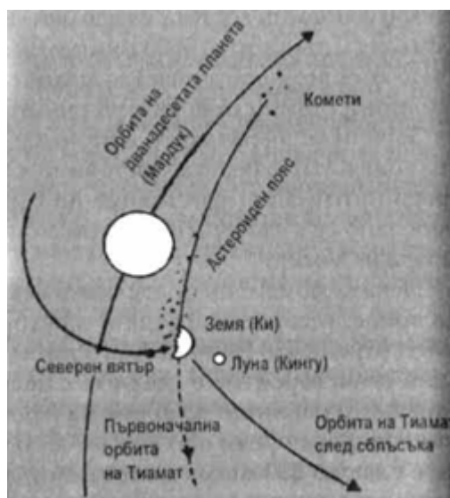
Изображение 32: Когато Нибиру/ Мардук прониква в нашата Слънчева система, променя орбитата на планетата Тиамат (първоначалната Земя). Една от луните на Нибиру се сблъсква с Тиамат и нарушава целостта ѝ. Откъснатата от нея част се отклонява от първичната си орбита, повлича една от двете луни на Нибиру и така възникват днешните Земя и Луна.
